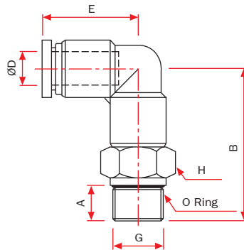
Metal Döner Dirsek / Metal Male Elbow
