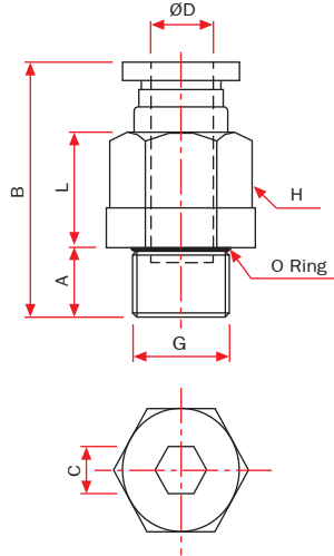
Metal Düz Rekor Erkek / Metal Male Straight
