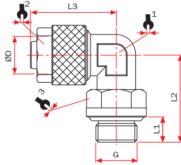
Metal Somun Sıkmalı Döner Dirsek / Metal Push on Fitting Male Elbow
